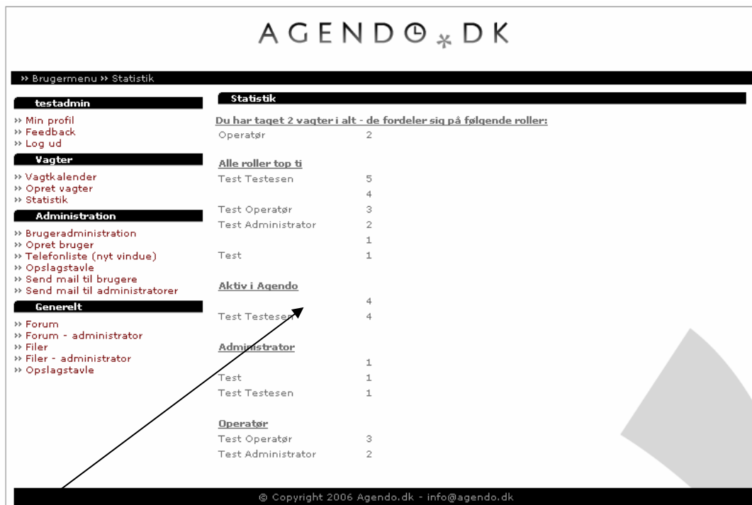
Fig. 4: Statistik
